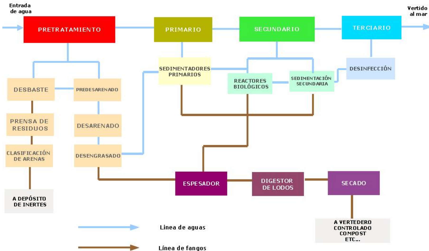
Diagrama de flujo del tratamiento de aguas residuales Memoria de Información Título V
