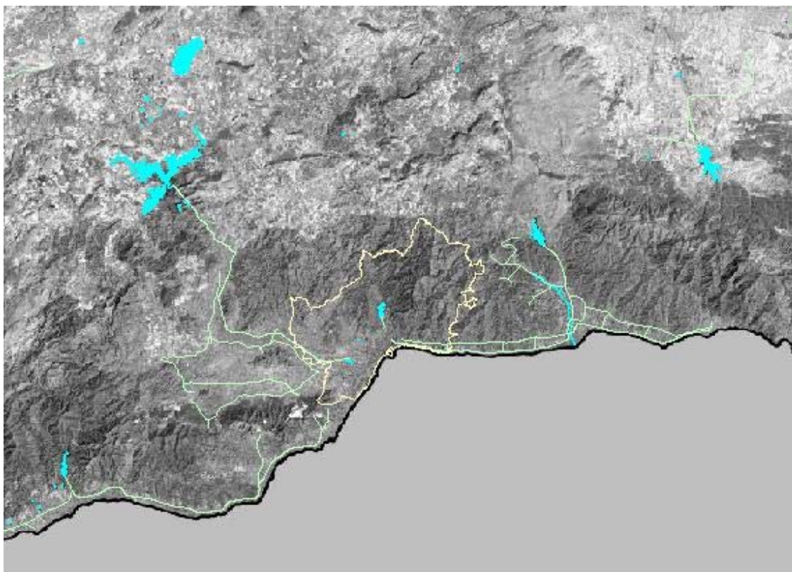
Imagen de los embalses suministradores y de la red de abastecimiento de Málaga
